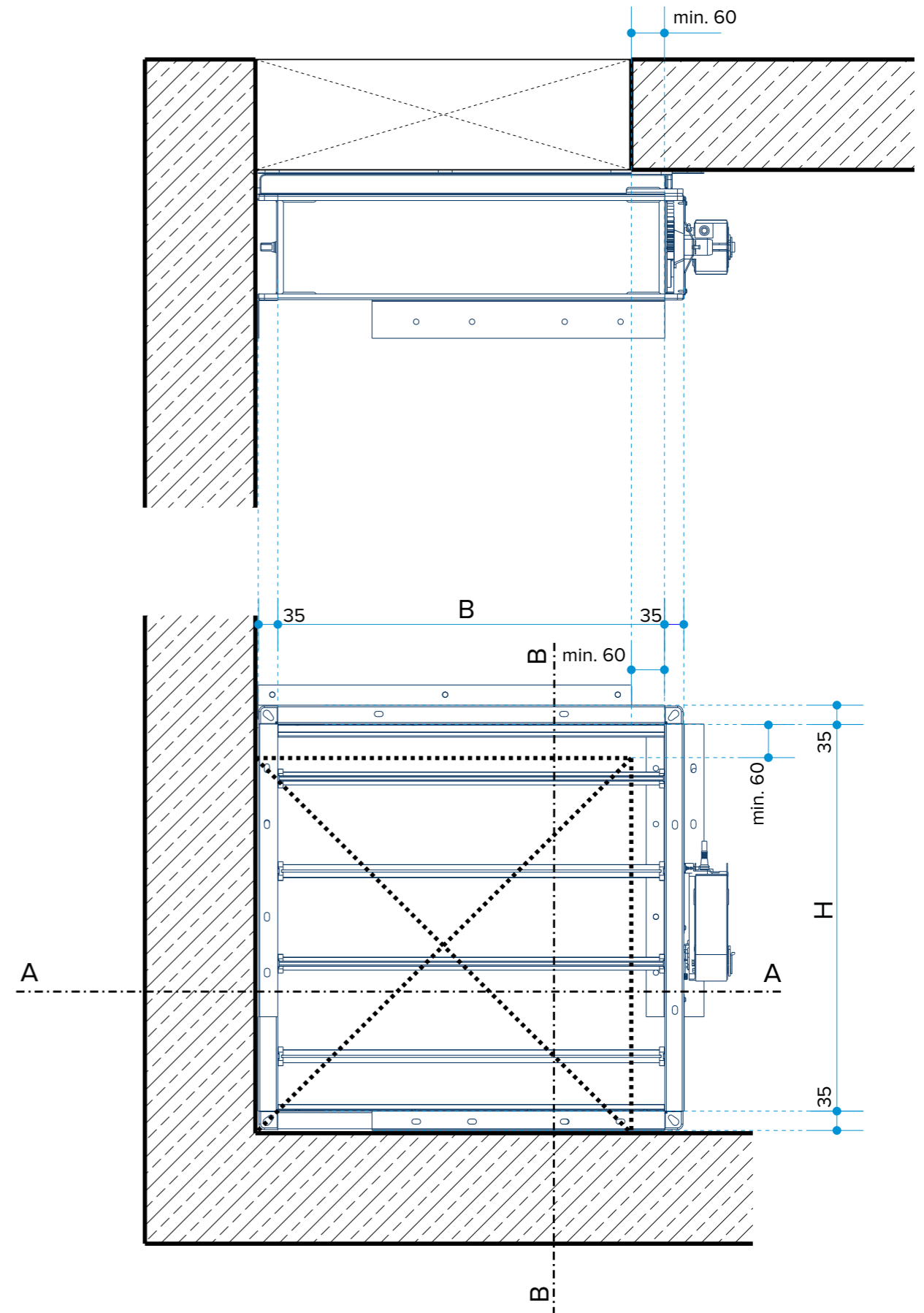
Schnitt A-A
