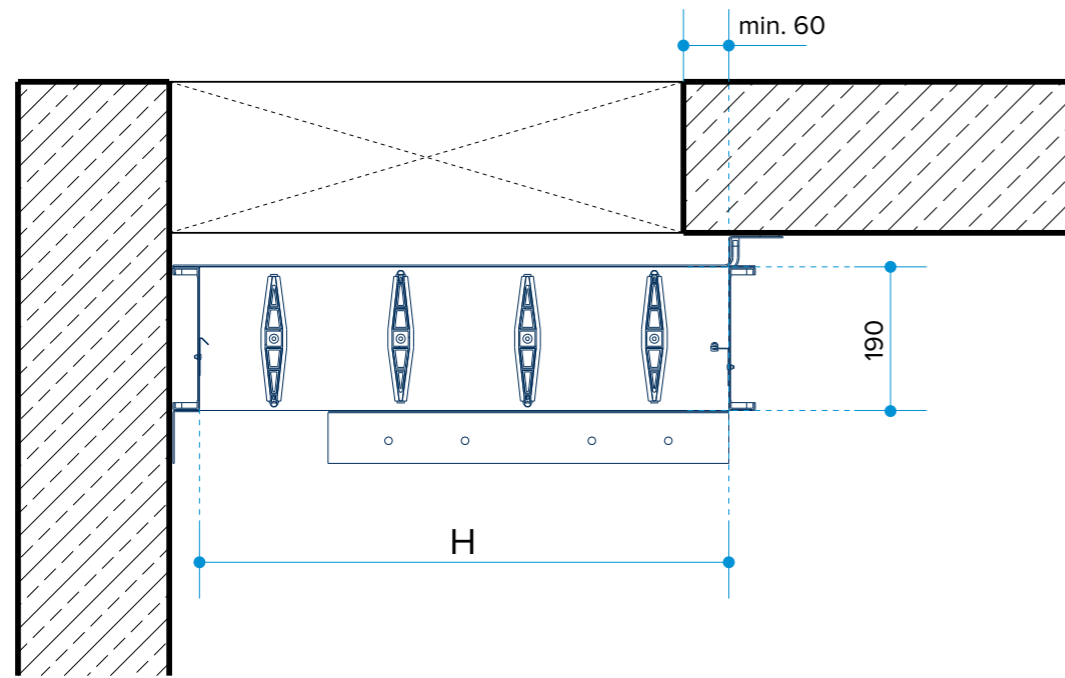
Schnitt B-B
